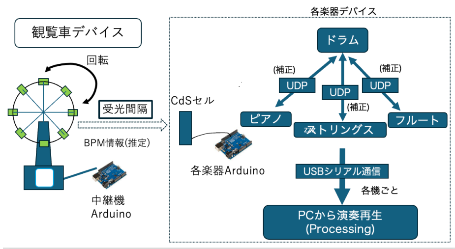
図 18 楽器デバイスのシステム構成図
